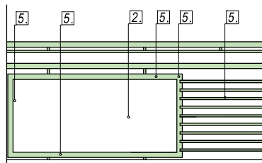
DETAL BALUSTRADY BAL.1 SKALA 1:50
