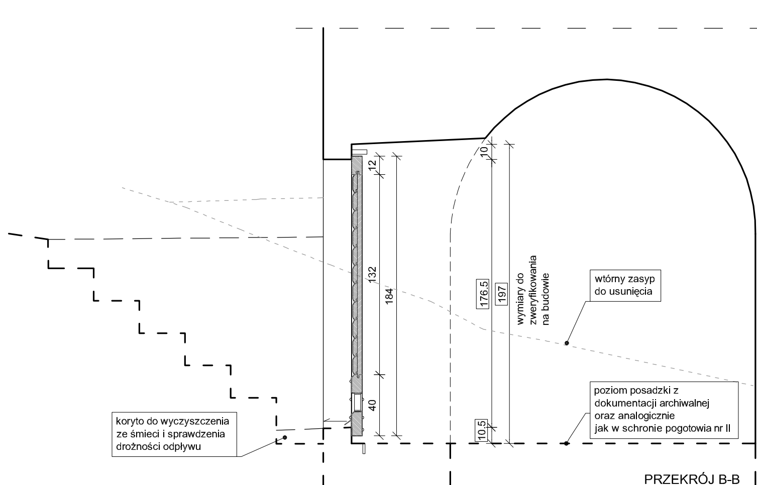
PRZEKRÓJ B-B OTWÓR sp7-o1
