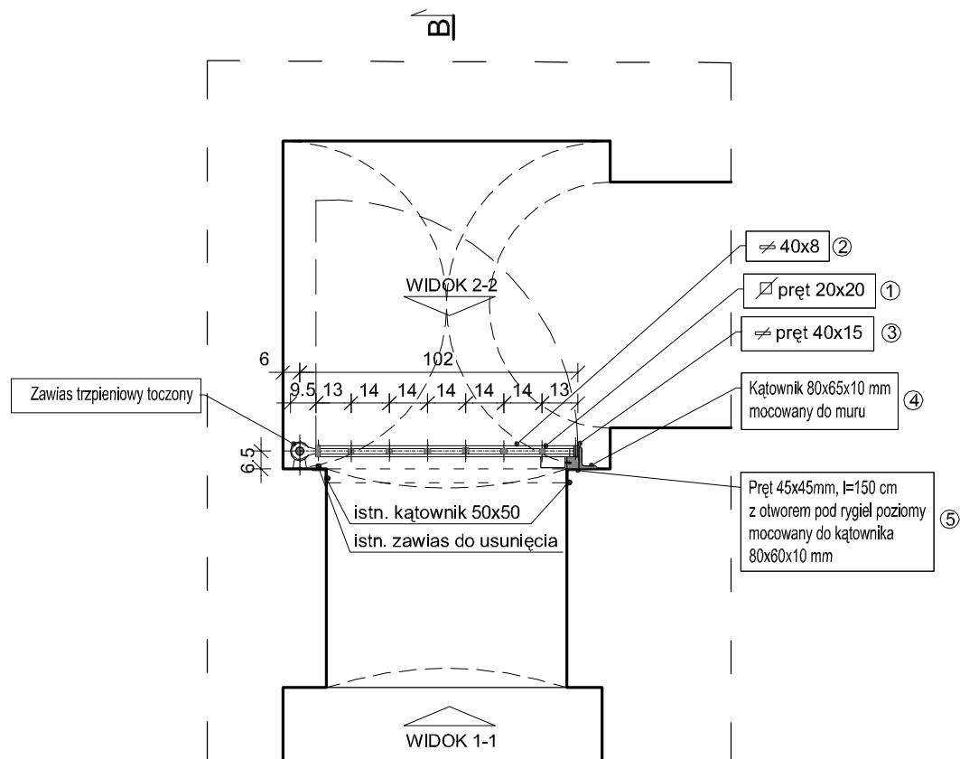
PRZEKRÓJ A-A OTWÓR sp7-o2
