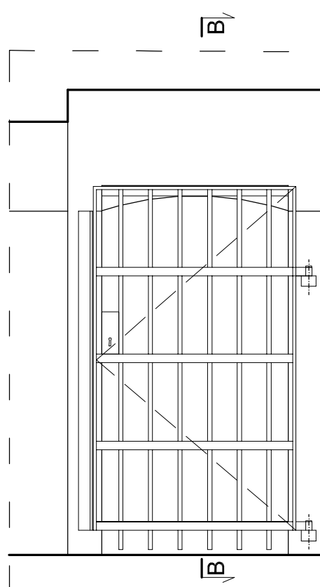
WIDOK OD WNEŹRZA 2-2 OTWÓR sp7-o2
