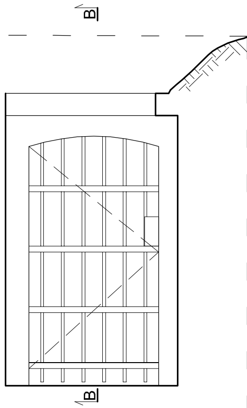
WIDOK OD STRONY ELEWACJI 1-1 OTWÓR sp7-o2
