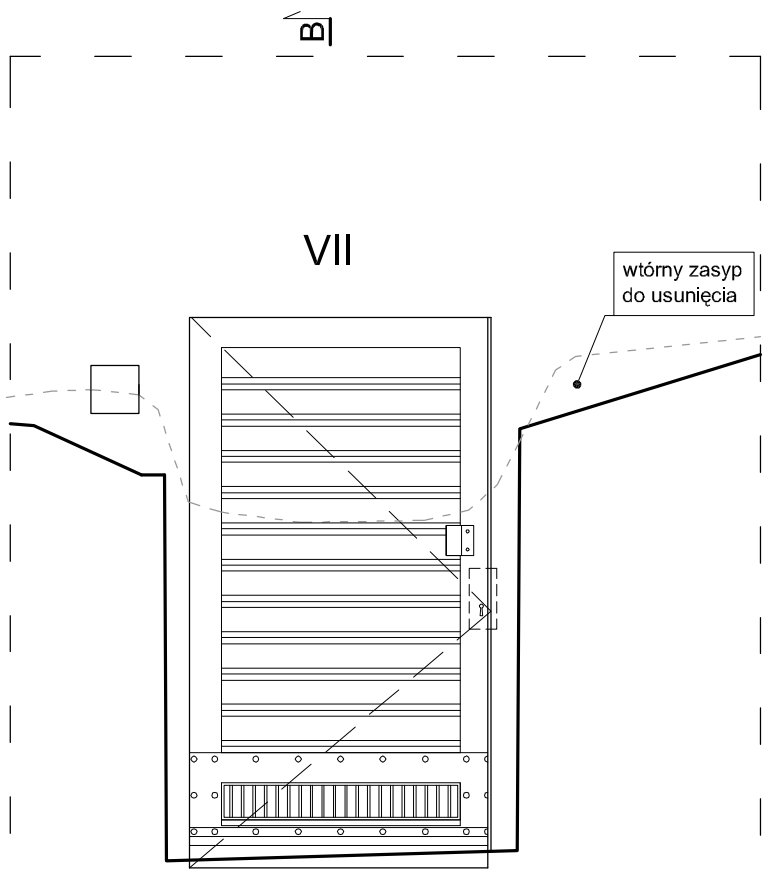
WIDOK OD STRONY ELEWACJI 1-1 OTWÓR sp7-o1
