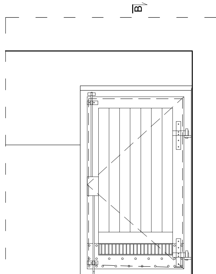
WIDOK OD WNEŹRZA 2-2 OTWÓR sp7-o1
