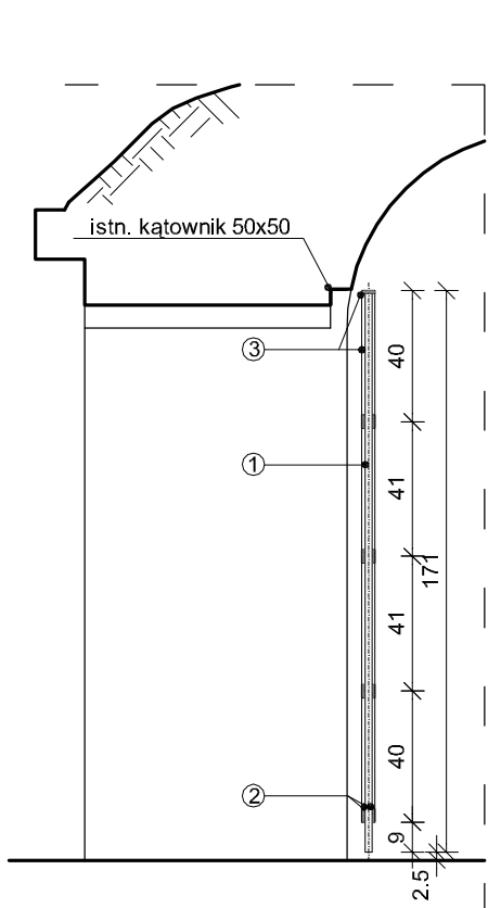
PRZEKRÓJ B-B OTWÓR sp7-o2
