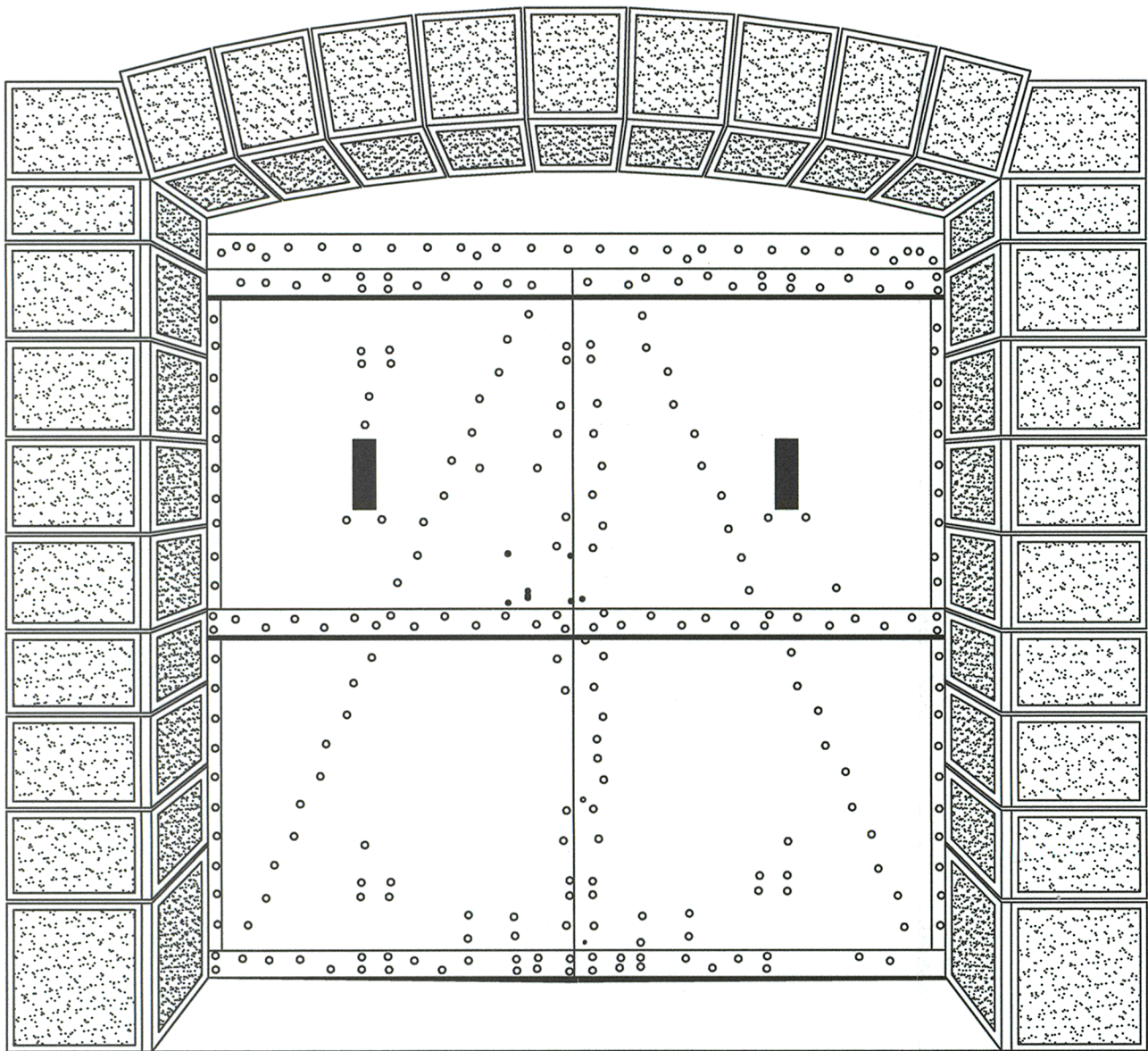
WIDOK PORTALU BRAMY GŁÓWNEJ KOSZAR – REKONSTRUKCJA UKŁADU OKŁADZINY TYNKOWEJ
