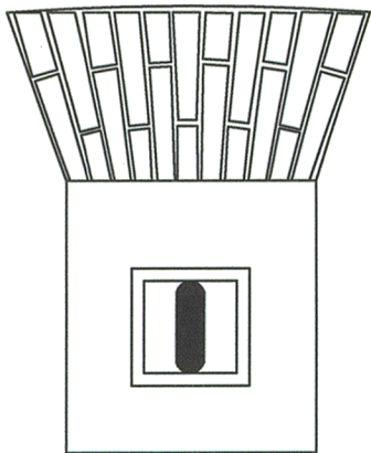
STRZELNICA SCHODKOWA KAPONIERY SZYJOWEJ WIDOCZNA CHARAKTERYSTYCZNA OPASKA BETONOWA, W GŁĘBI PŁYTA PANCERNA
