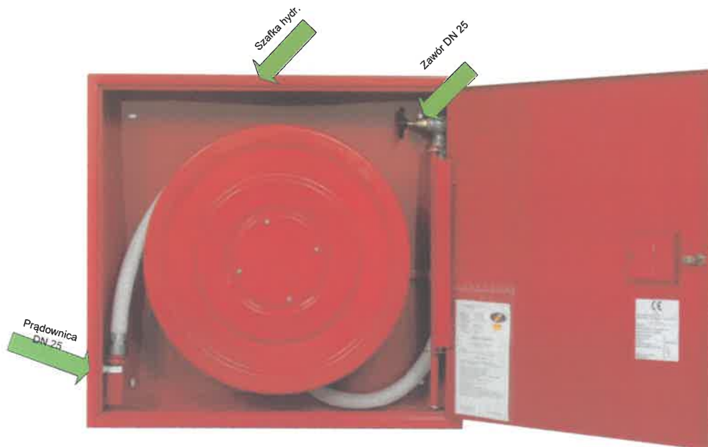
Hydrant wewnętrzny 25 z węzem półsztywnym
