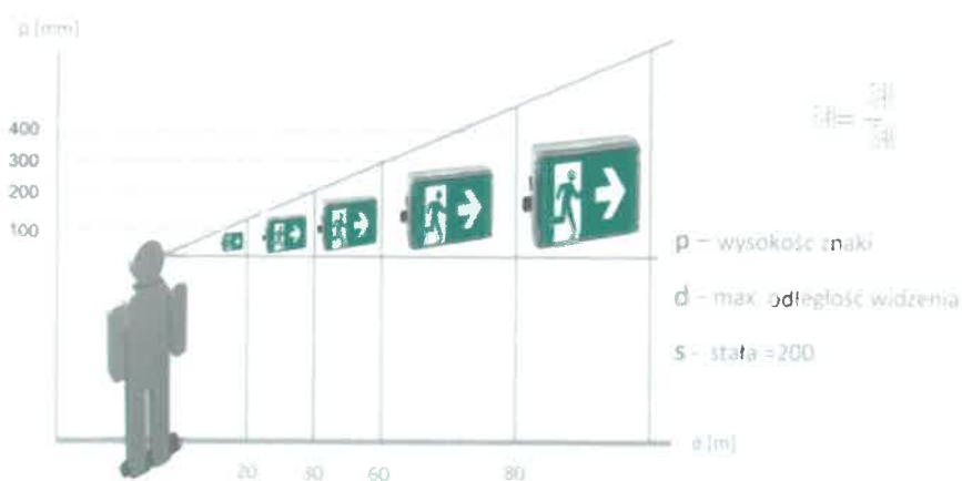
Rysunek nr 2. Znaki oświetlone: wewnętrznie: stała s = 200
