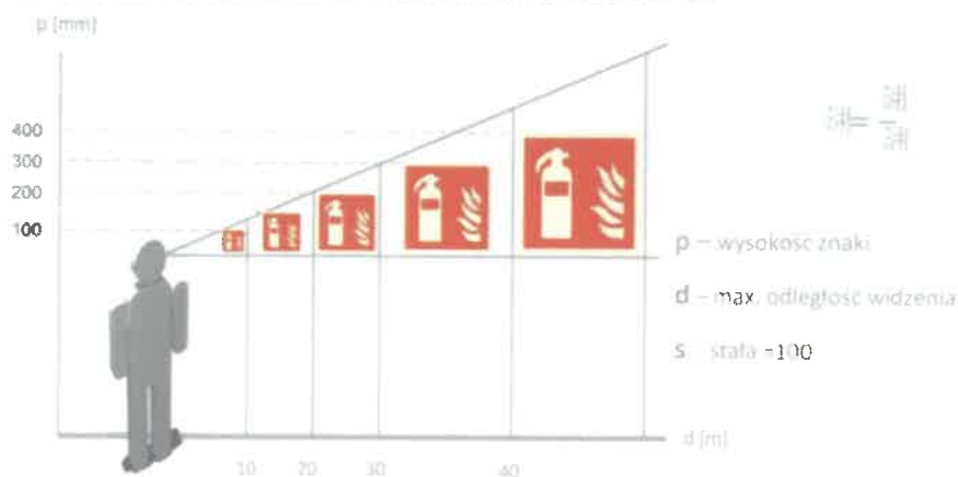
Rysunek nr 1. Znaki USA: wewnętrzne: stała s = 100
