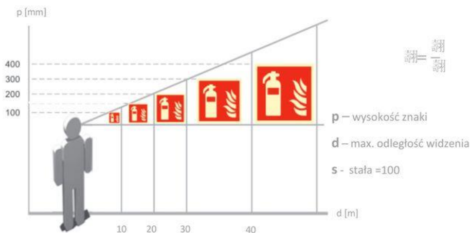
Rysunek nr 1 . Znaki oświetlone zewnętrznie stała s = 100 .
